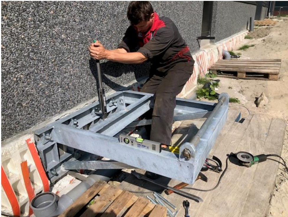
montage mast-bok aan fundering
